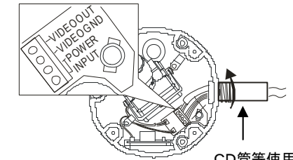
図4.配線図
