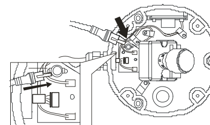
図7.調整用出力端子
