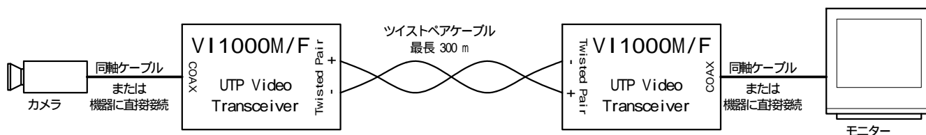
接続図
